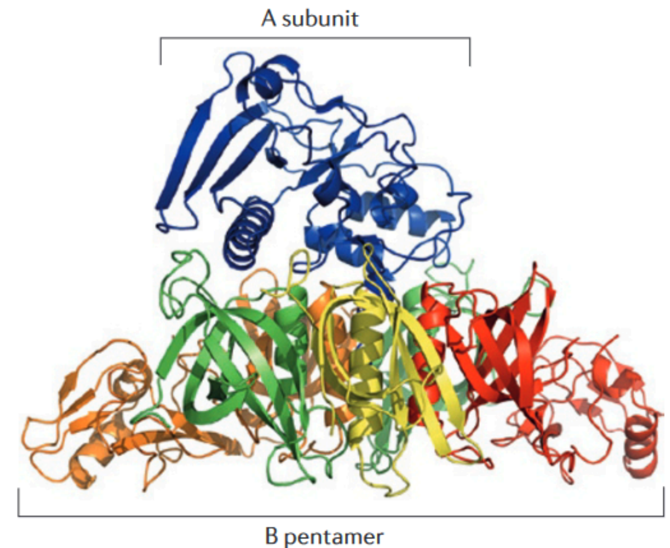
Structure de la toxine pertussique
